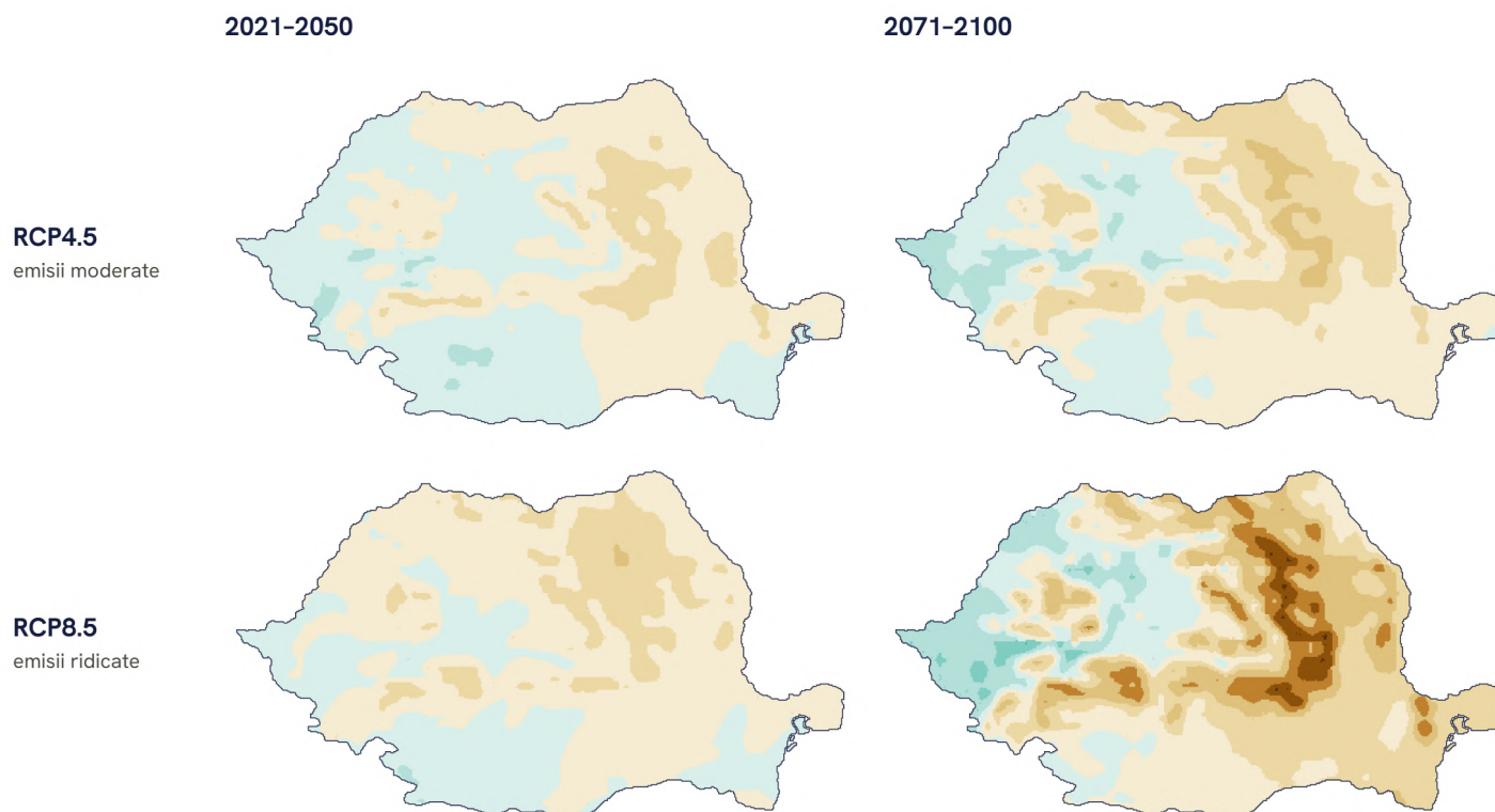
Figura 8. Anomalii estimate pentru deficitul de apă din sol la nivelul României, pentru orizonturile 2021–2050 și 2071–2100, în scenariile RCP4.5 și RCP8.5.
