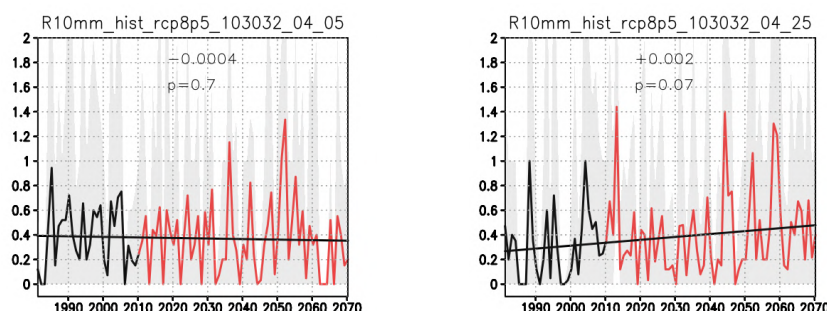
Figura 9. Indicele R10: numărul de zile cu precipitații peste 10 mm/zi, media pe decadă, pentru prima și ultima decadă a lunii aprilie (analizat pentru sudul țării).
