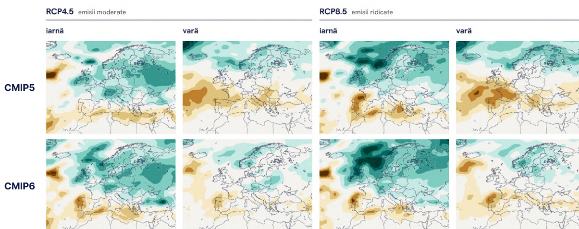
Figura 3. Abateri estimate pentru precipitațiile totale, în scenariile CMIP6 față de CMIP5, pentru forță radiativ echivalent RCP4.5 și RCP8.5.
