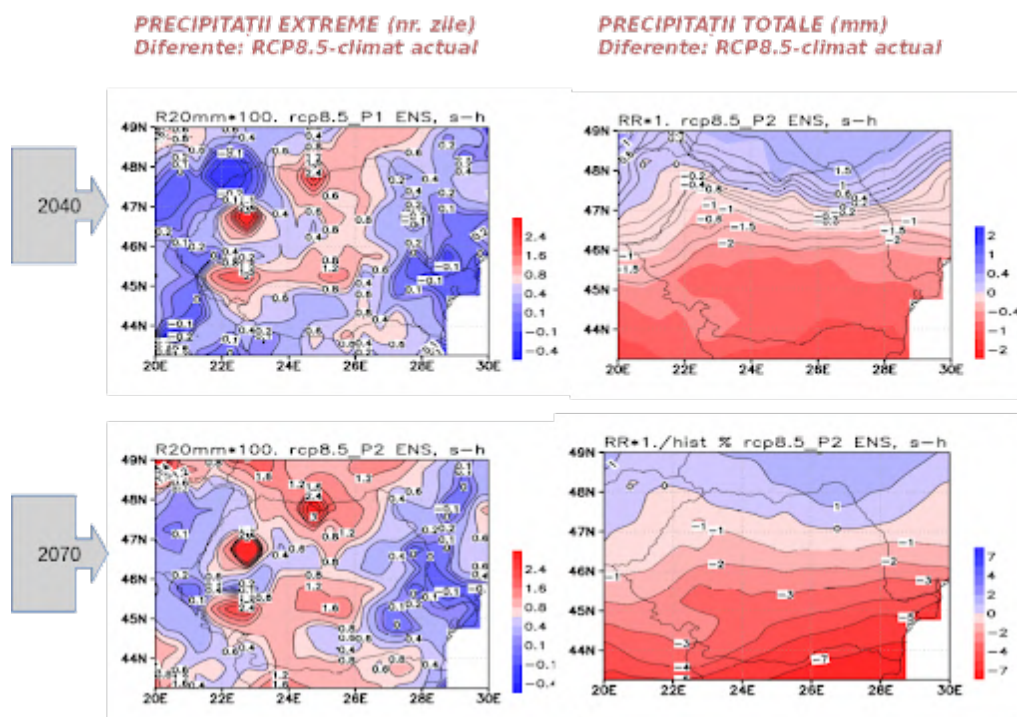
Figura 10. (stanga): abateri în numărul zilelor cu precipitații de peste 20 mm/zi (Indicele R20) dintr-un interval de zece zile, medie pe 30 de ani, multi-model, RCP8.5 (orizont 2040 sus și 2070 jos); (dreapta): abateri în precipitațiile totale pentru RCP8.5, orizont 2070: valori absolute (sus) și procente (jos).
