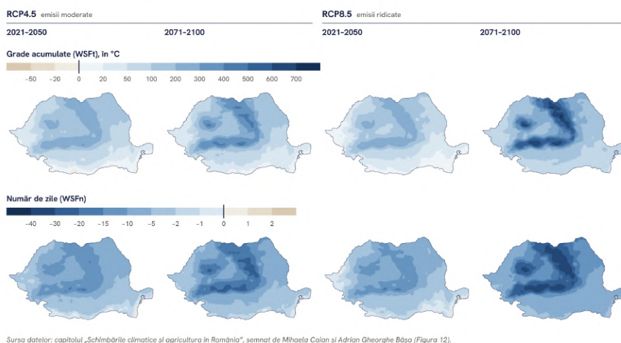
Figura 12. Indicele de îngheț sever de iarnă WSF
