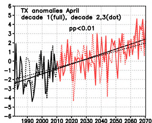
Figura 15. Tendința de creștere a temperaturii maxime diurne (TX), semnificativă statistic, în proiecții climatice multi-model pentru aprilie, pe cele trei decade (exemplu pentru sudul țării).
