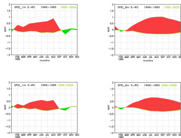
Figura 4. Intensificarea secetei meteorologice în ultimele decenii în România: Indicele SPEI lunar : Est – Moldova și Dobrogea (sus) și Sud – Oltenia și Muntenia (jos), calculat din date Copernicus pentru deceniile 1966-1995 (negru) versus 1996-2025 (verde). Figura arată creșterea indicelui de secetă SPEI în ultimele decenii, maxima în august, urmată de toamne mai umede în deceniile recente.
